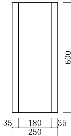
180*600 U型溝
