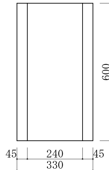
240*600 U型溝
