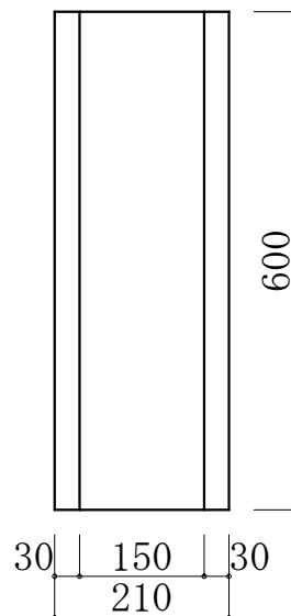
150*600 U型溝
