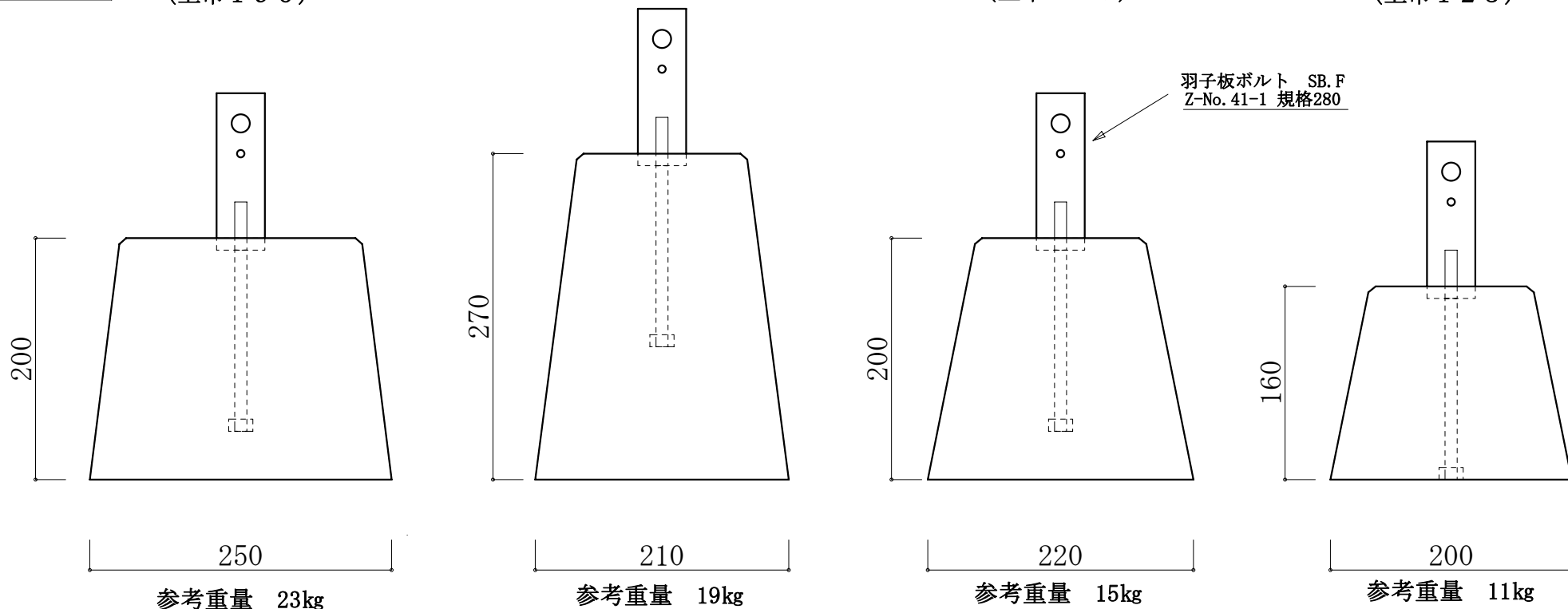
側面図
