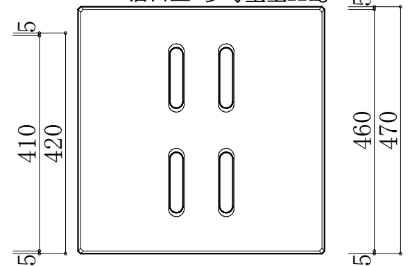
400 溜桝蓋 参考重量22kg
