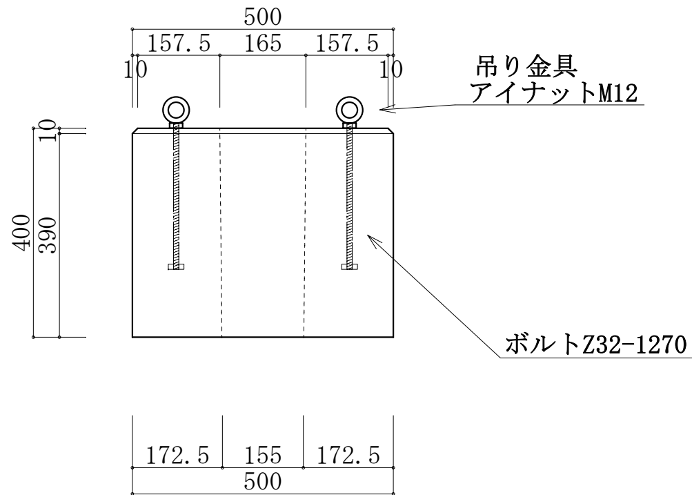
側面図
