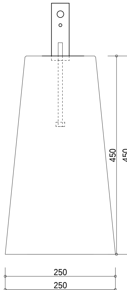
側面図
