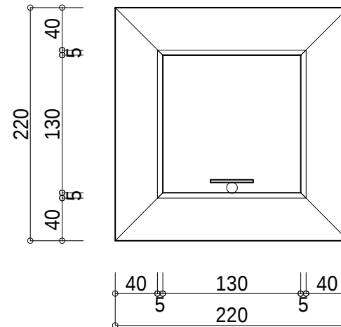
3 寸柱用羽子板束石H=200 ( 上巾 1 3 0 )
