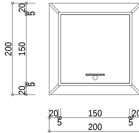
4 寸柱用羽子板束石H=200 ( 上巾 1 5 0 )
