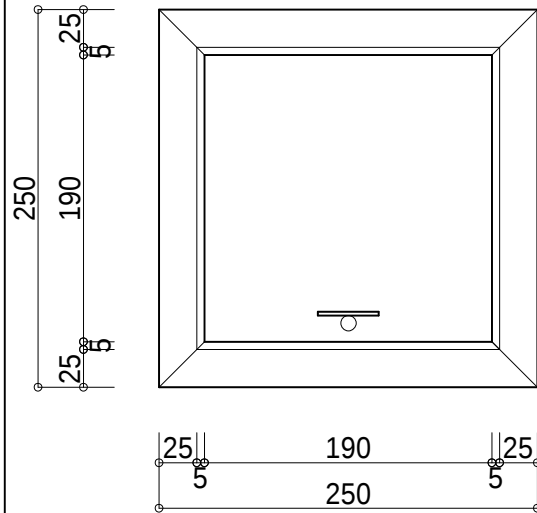
5 寸柱用羽子板束石H=200 ( 上巾 1 9 0 )
