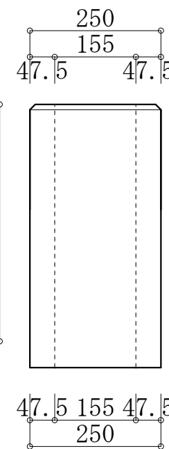
250*500 フェンス基礎石
