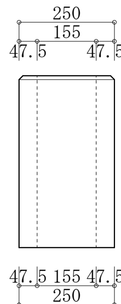
250*450 フェンス基礎石
