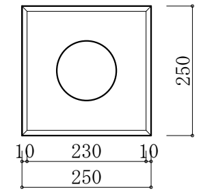
250*250 フェンス基礎石
