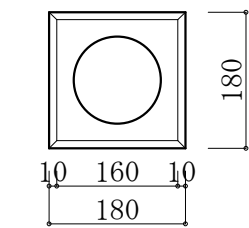
180*450 フェンス基礎石
