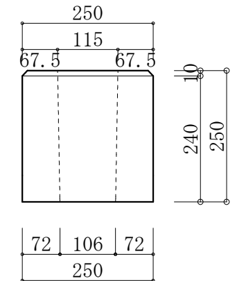
250*250 フェンス基礎石
