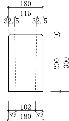
180*300 フェンス基礎石
