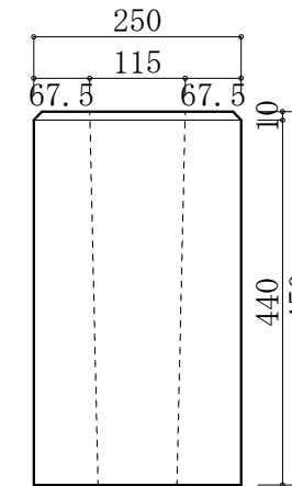
250*450 フェンス基礎石
