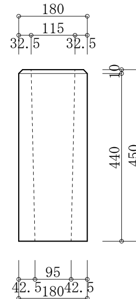
180*450 フェンス基礎石
