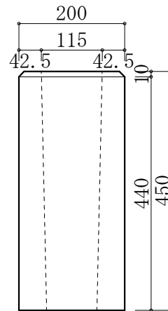
200*450 フェンス基礎石
