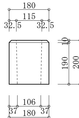
180*200 フェンス基礎石
