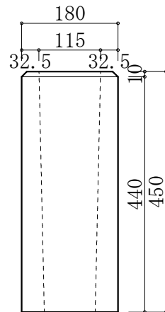
180*450 フェンス基礎石
