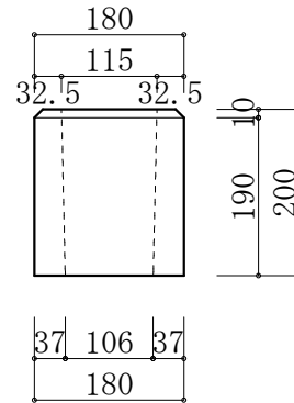
180*200 フェンス基礎石
