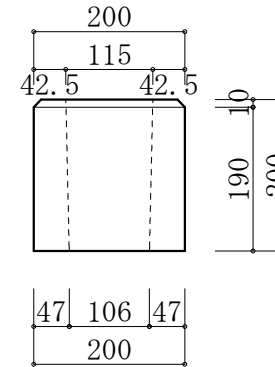
200*200 フェンス基礎石
