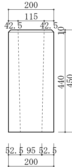
200*450 フェンス基礎石
