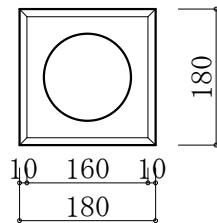
180*450 フェンス基礎石
