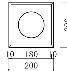
200*200 フェンス基礎石
