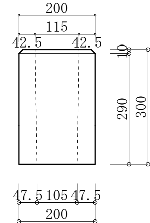
200*300 フェンス基礎石
