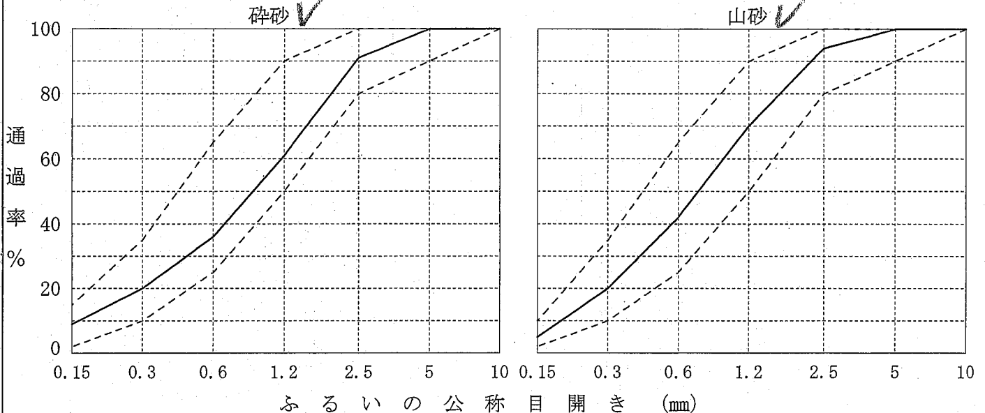
粒 度 曲 線
