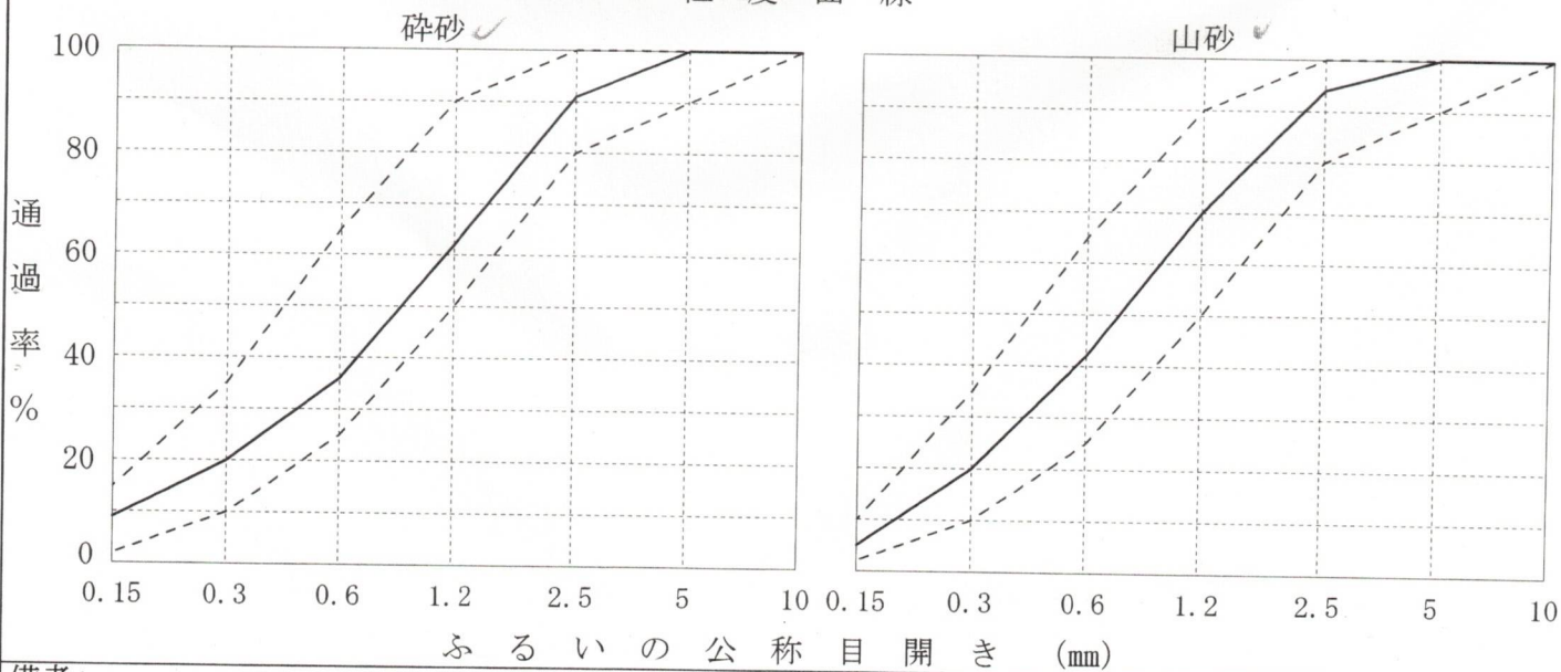
粒度曲線
