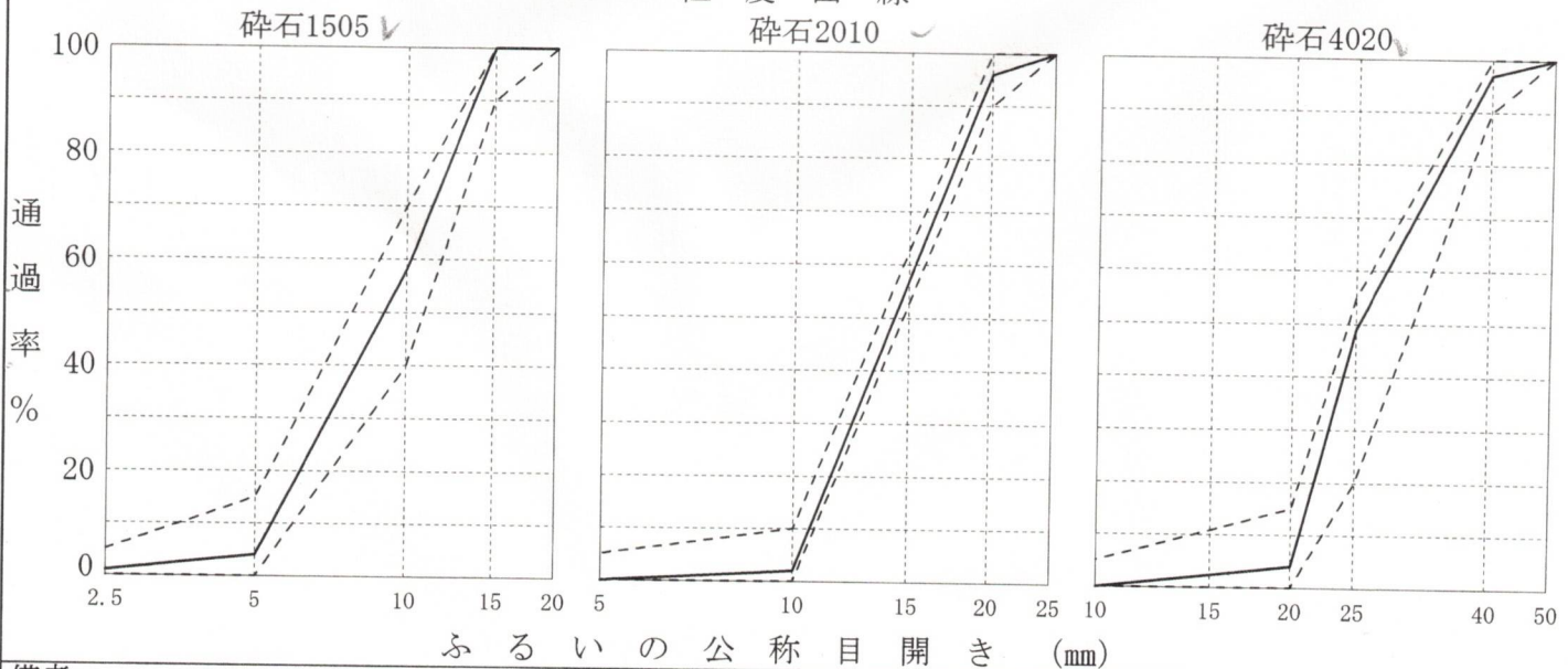
粒 度 曲 線
