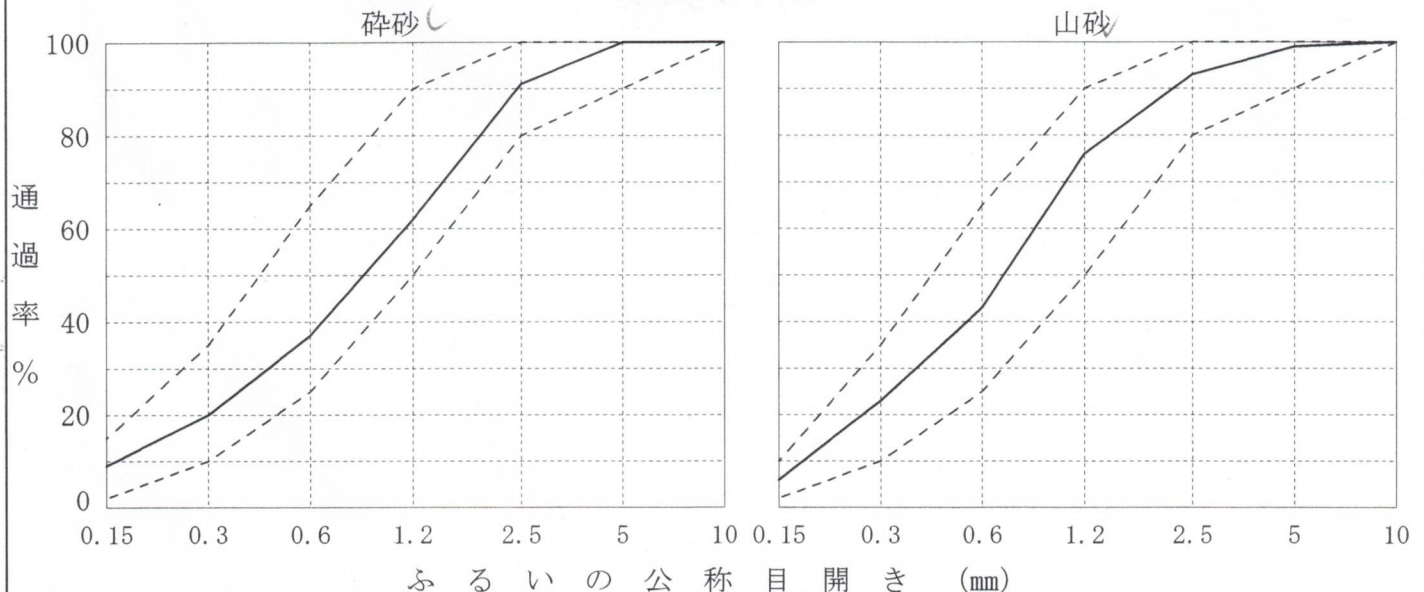
粒 度 曲 線
