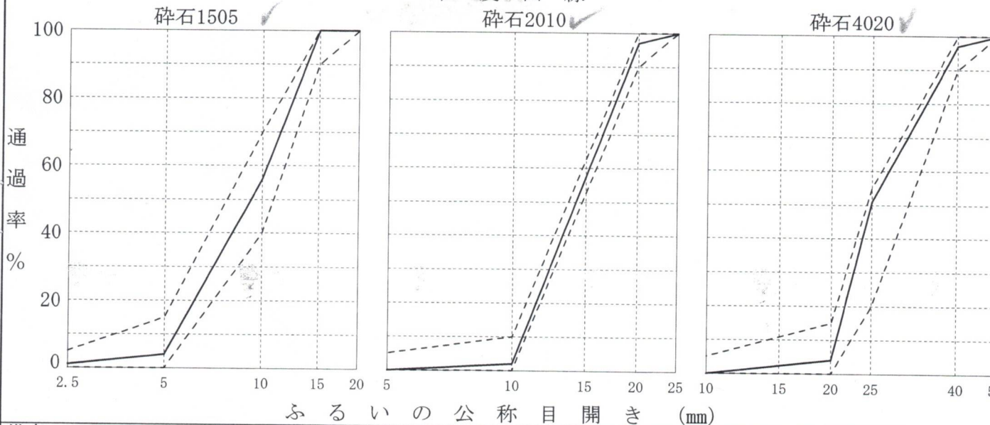
粒度曲線
