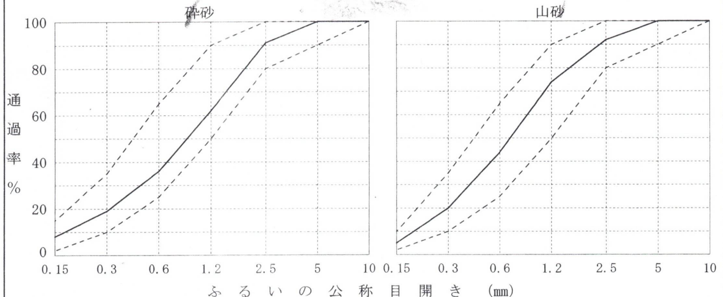
粒 度 曲 線
