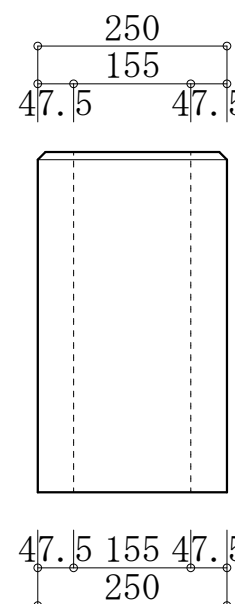
250*450 フェンス基礎石
