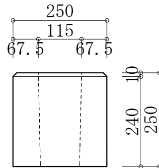
250*250 フェンス基礎石
