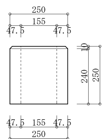
250*250 フェンス基礎石
