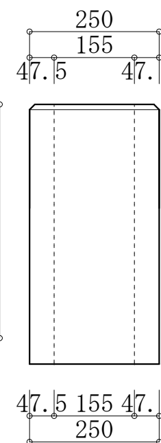
250*500 フェンス基礎石
