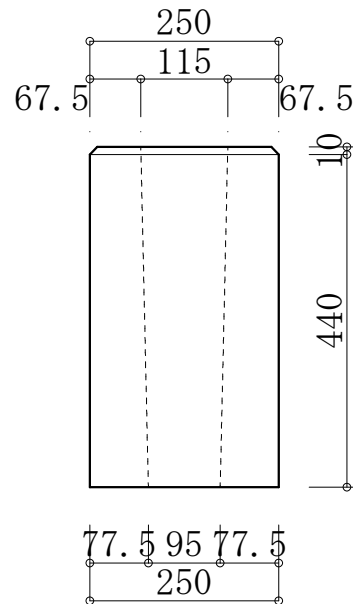
250*450 フェンス基礎石
