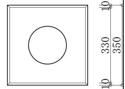
350*600基礎石 参考重量 140Kg
