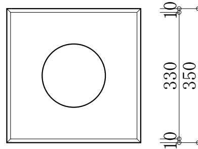
350*250基礎石 参考重量 58Kg
