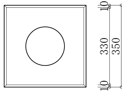
350*200基礎石 参考重量 47Kg
