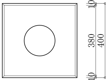
400*400基礎石 参考重量 122Kg
