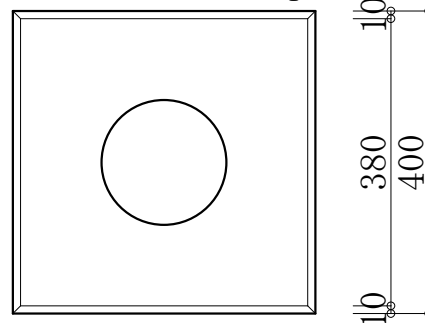
400*500基礎石 参考重量 150Kg
