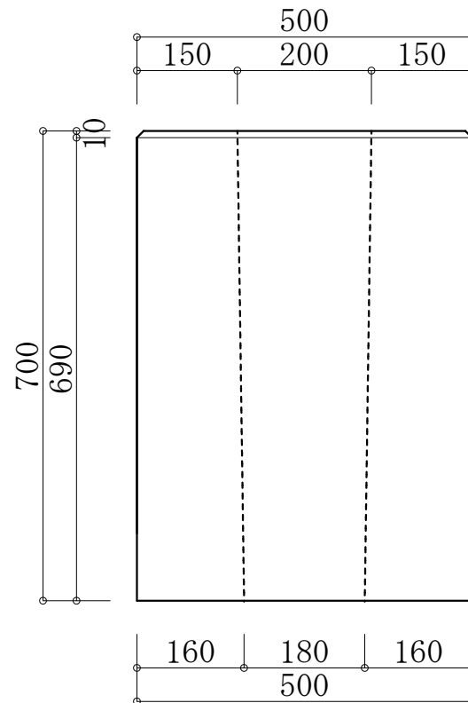
側面図
